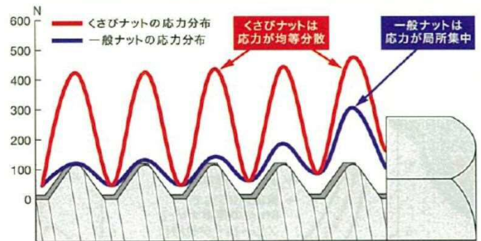
くさびナットねじ部
