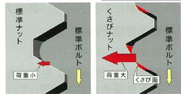
くさびナットねじ部
