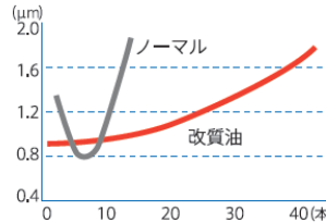
真円度測定結果
