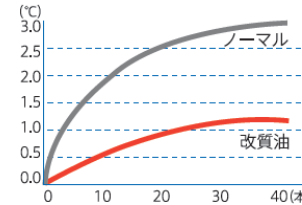
被削材温度測定結果
