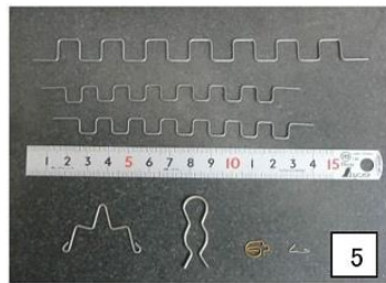
3~5. トーションバネ 線径φ0.2~φ2.0 丸線曲げ加工線径φ0.5~φ6.0
