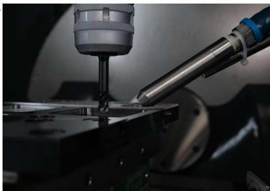
ドライアイスパウダー クーラントシステム D I P S
