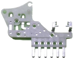
POM材+金属インサート
