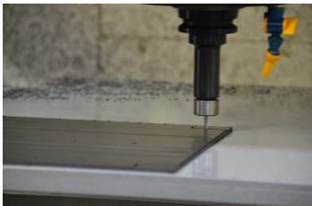
試作 (切削・ウォータージェット加工)
