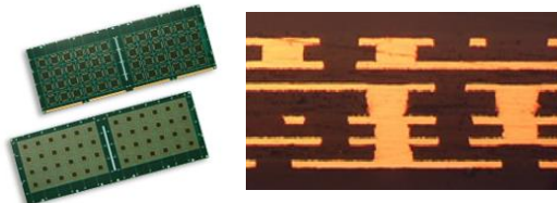
(半導体パッケージ用基板 6層2-2-2 Build Up)
