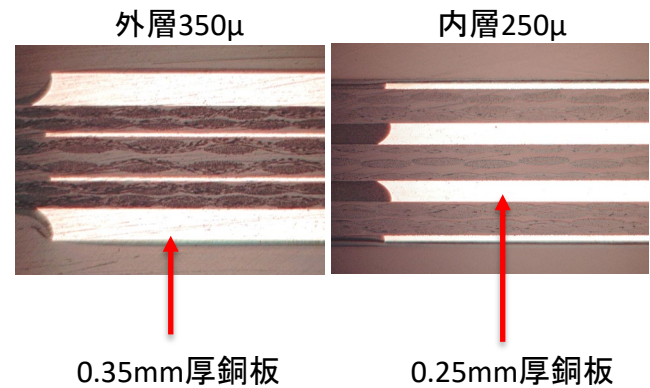
大電流対応基板の断面図
