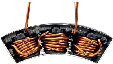
分割コア巻き 連続コイル
