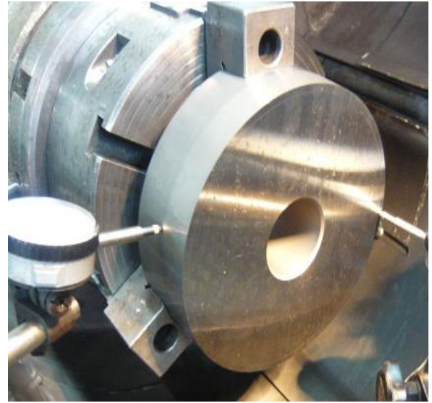
転造盤用 ロールダイス製作(ツガミ殿向け)
