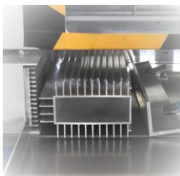
・アルミ型材切断機
