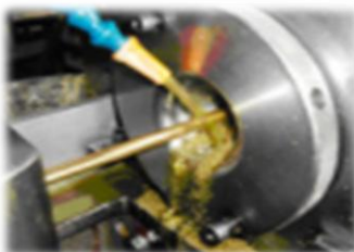
・引抜ローレット加工機
